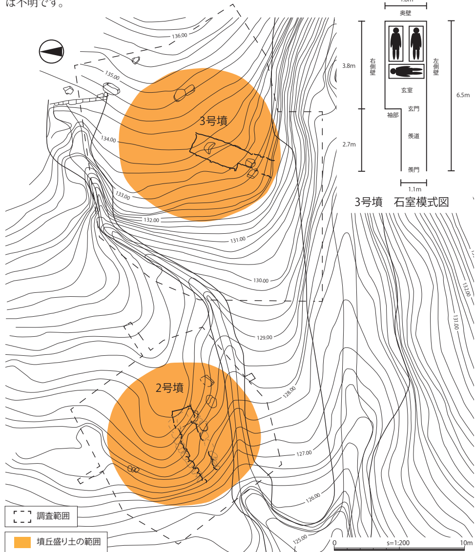
福林寺古墳群遺構配置図(S=1/200)
