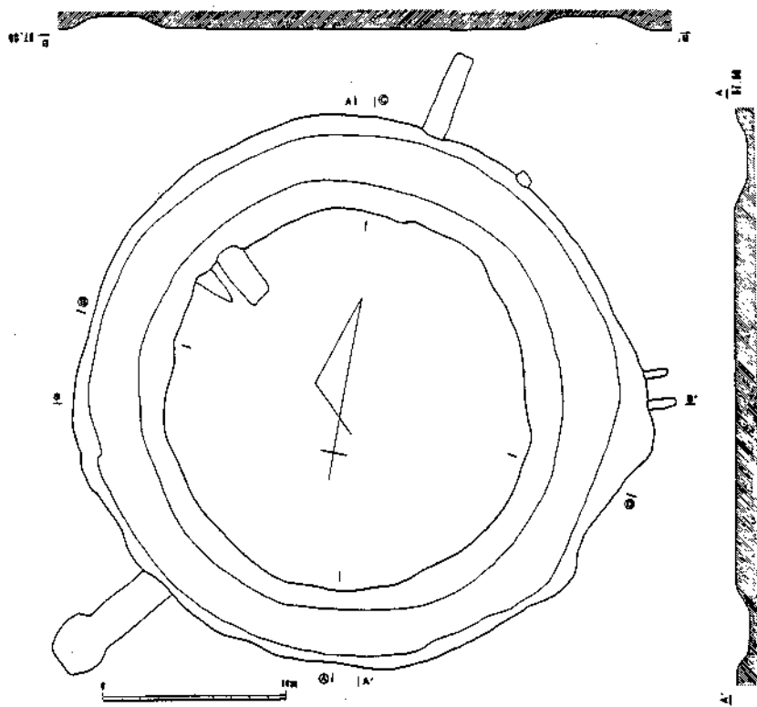
服部遺跡23号墳平面実測図
